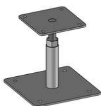
Platine réglable Inox 100x100/130x130mm épais. 4mm
